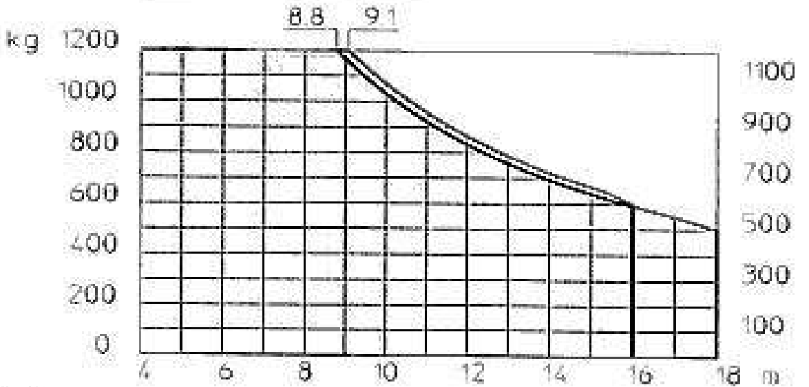
DIAGRAMMA DI CARICO
