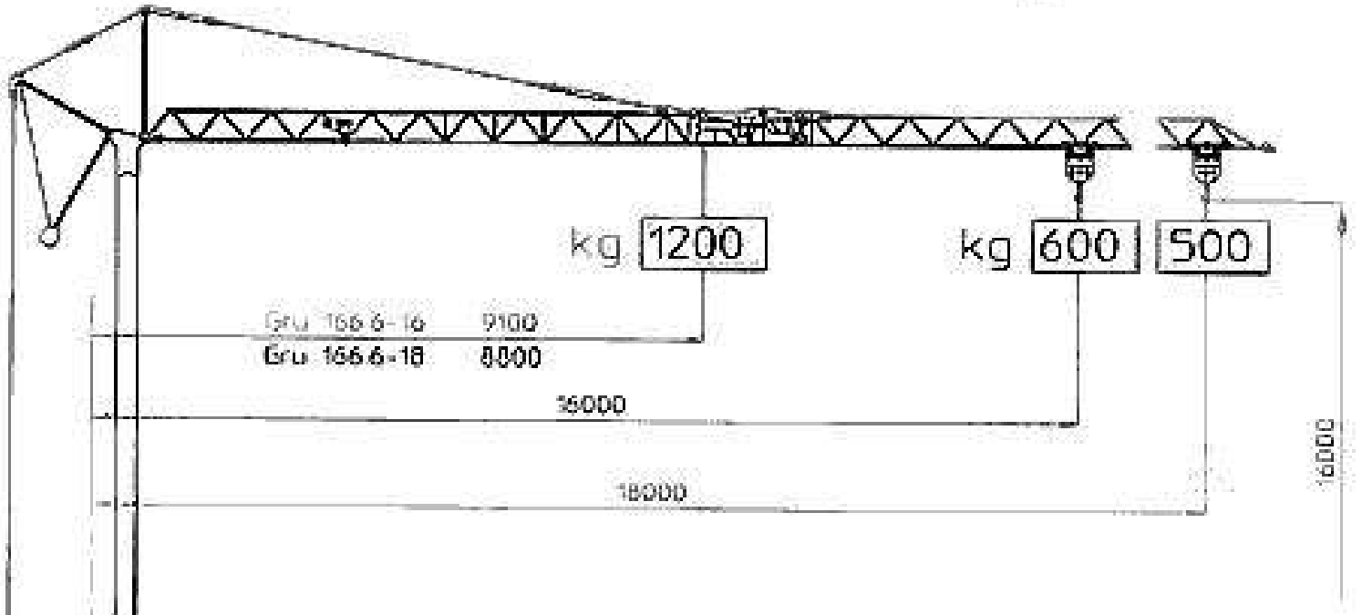
DIAGRAMMA DI CARICO
